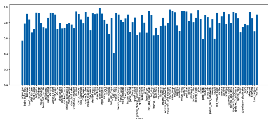
Figura 8. F1 media por cada clase para ResNet50.
