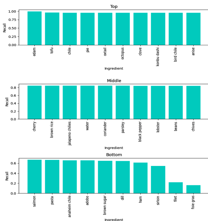
Figura 6. Mejores, medios y peores ingredientes reconocidos con el modelo ML-AFM.
