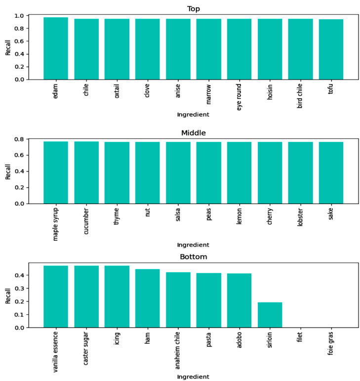
Figura 5. Mejores, medios y peores ingredientes reconocidos con el modelo ResNet50.
