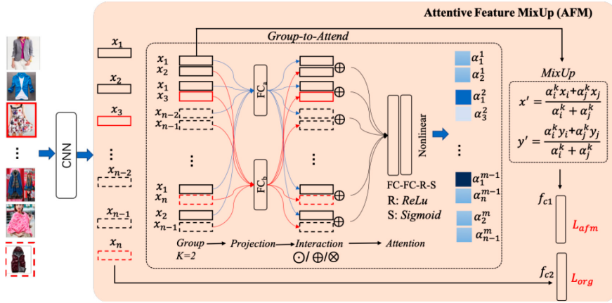
Figura 1. Flujo de proceso del método AFM propuesto para la clasificación de etiqueta-única en muestras ruidosas [37].
