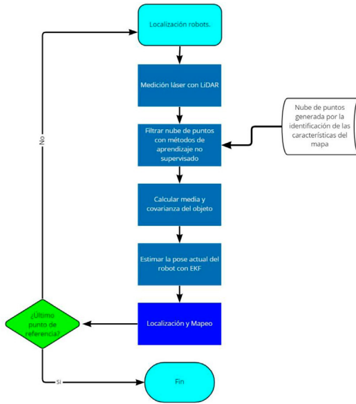
Figura 2. Diagrama de Flujo del sistema propuesto para la localización y mapeo del robot.
