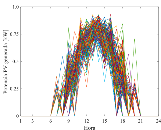
Figura 2. Curvas de generación FV-verano.
